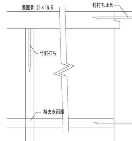
コーナー及び中骨組図 1:2
