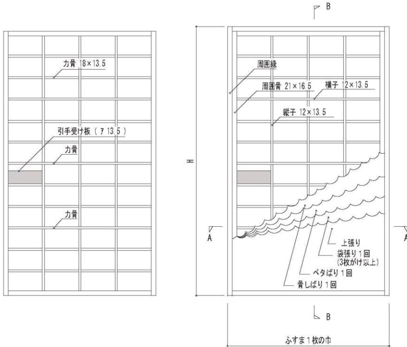
骨組図 1:15
