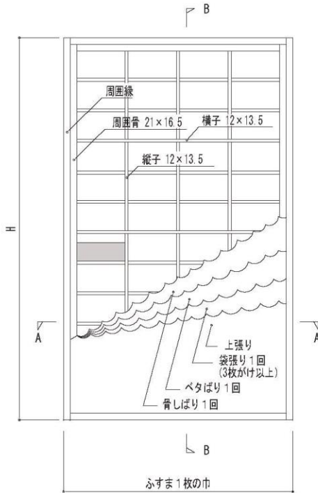
姿図 1:15
